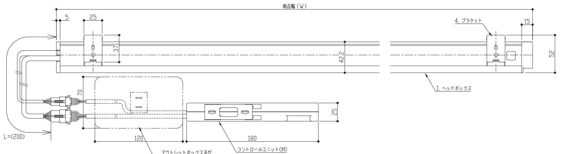
伏図
