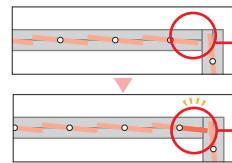
●コーナー窓仕様(ルーバー幅100mmのみ対応)
